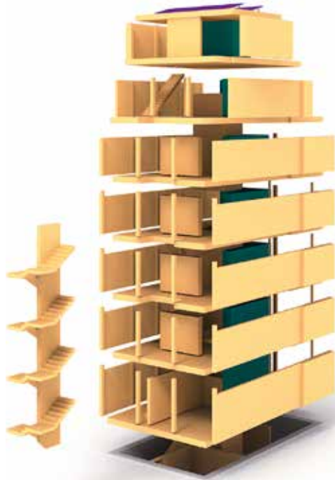
Abb. unten_Konstruktionsprinzip eines hochgradig vorgefertigten Elementbaus.
